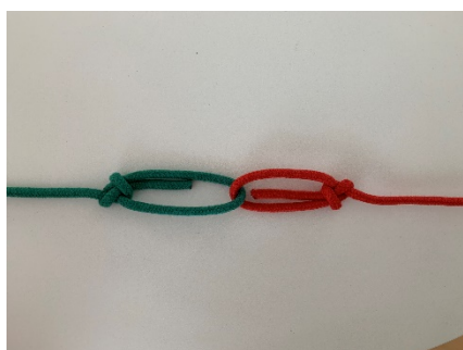
Pælestik (Deltager 1 og 2)
